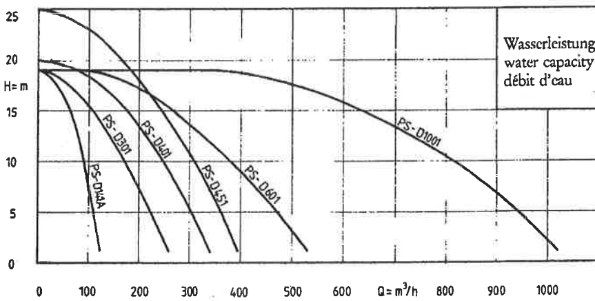
Leistungskurven
