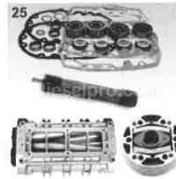
8V92 Blower - Turbo ( https://dieselpro.com/detroit-diesel-blower-53-71-92-149-series/8v92-blower-for-turbo )
