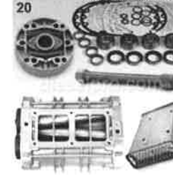
16V71 Blower - Non-Turbo ( https://dieselpro.com/detroit-diesel-blower-53-71-92-149-series/16v71-blower.html )
